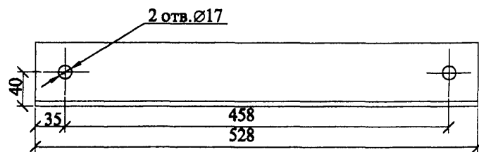
Поз. 3
