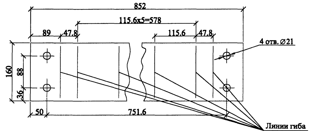
Развёртка поз. 5
