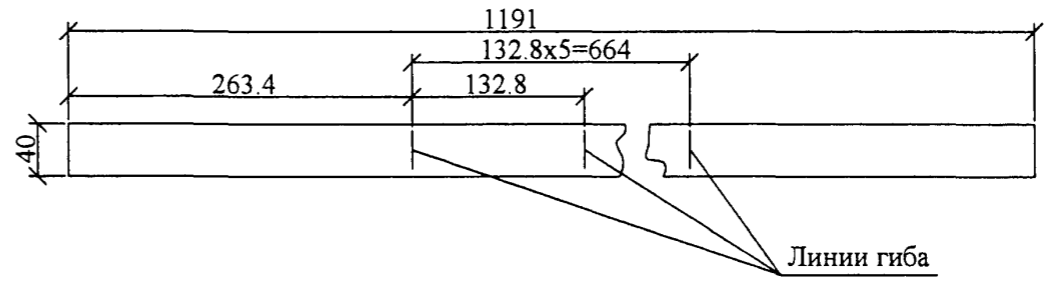
Развёртка поз. 1
