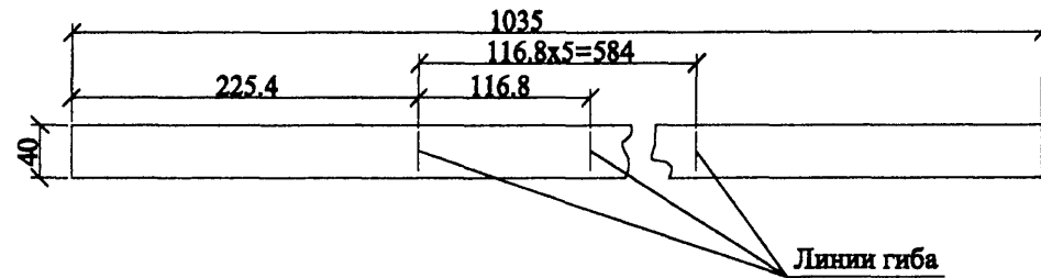
Развёртка поз. 1
