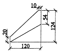
Поз. 2
