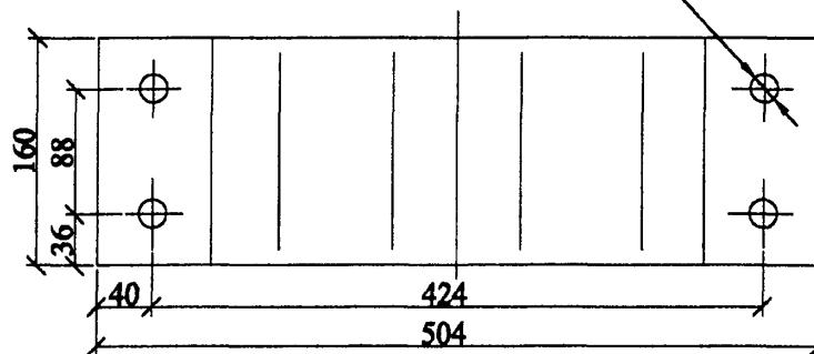
4 отв. Ø21
