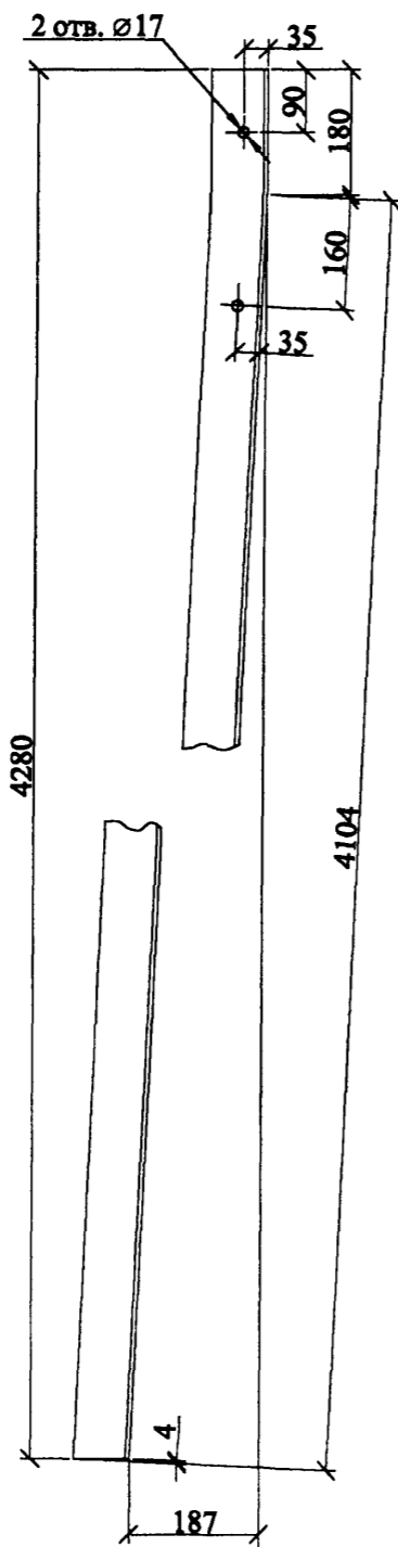
Поз. 2
