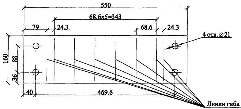
Развёртка поз. 3
