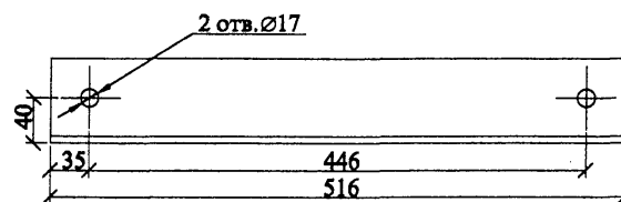
Поз. 3
