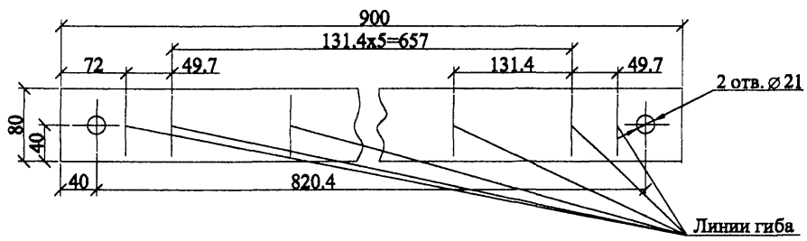
Развёртка поз. 1
