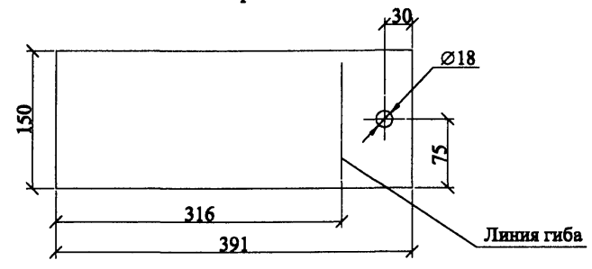
Развёртка поз. 1
