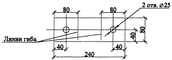
Поз. 3
