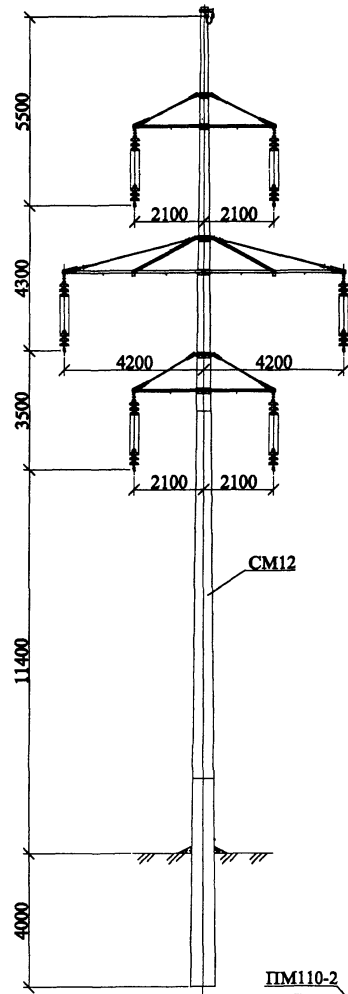
Двухцепная промежуточная опора ПМ110-2
