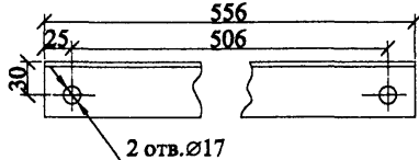
Поз. 1
