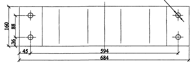
4 отв. Ø21
