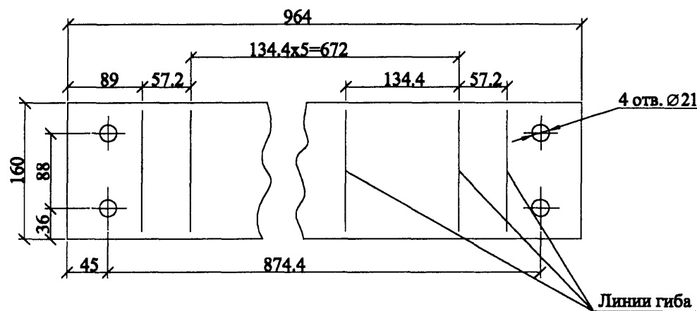
Развёртка поз. 4
