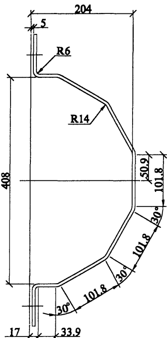
Поз. 4
