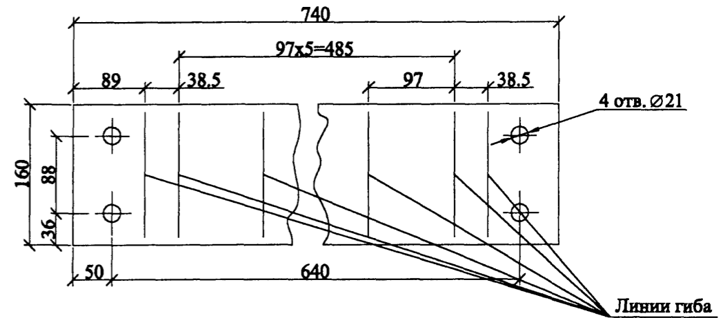
Развёртка поз. 7
