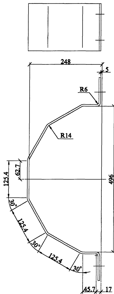
Поз. 4
