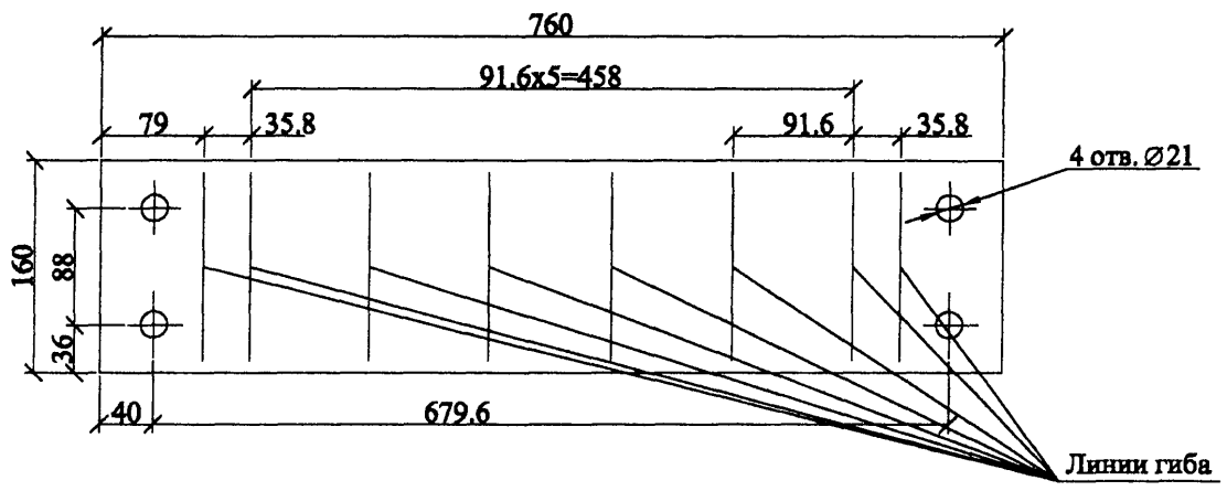
Развёртка поз. 5
