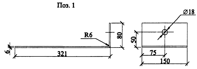
Развёртка поз. 1
