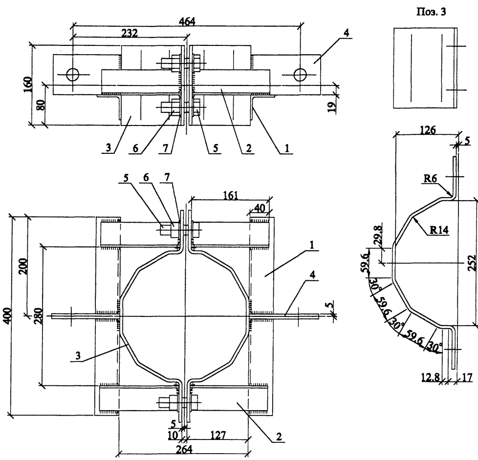
Развёртка поз. 3
