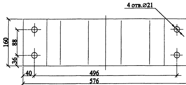
Развёртка поз.3
