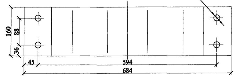
4 отв. Ø21
