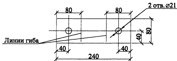
Поз. 3
