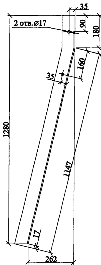
Поз. 2
