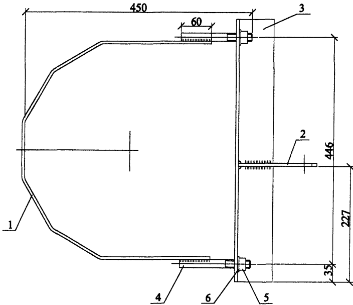
Поз. 2
