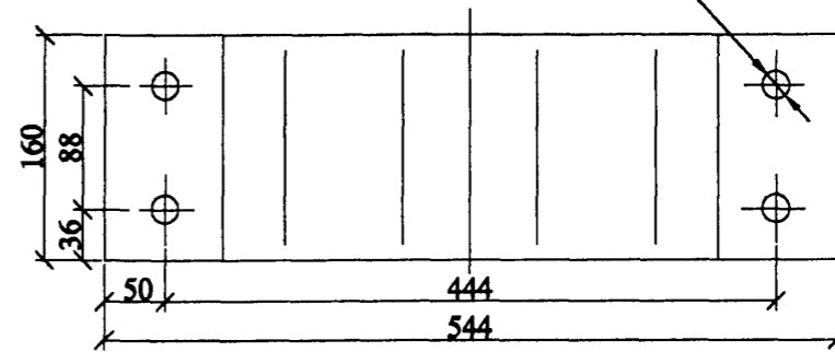
4 отв. Ø21
