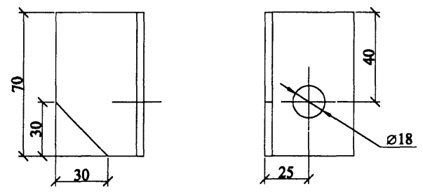
Поз. 2
