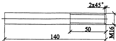
Поз. 4
