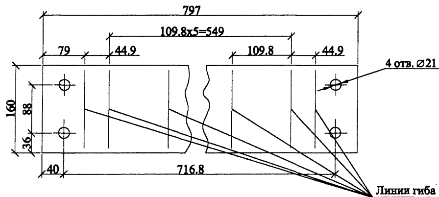
Развёртка поз. 3
