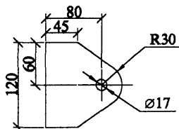
Поз. 4
