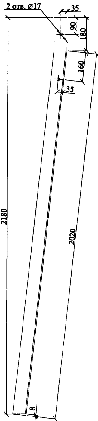
Поз. 2
