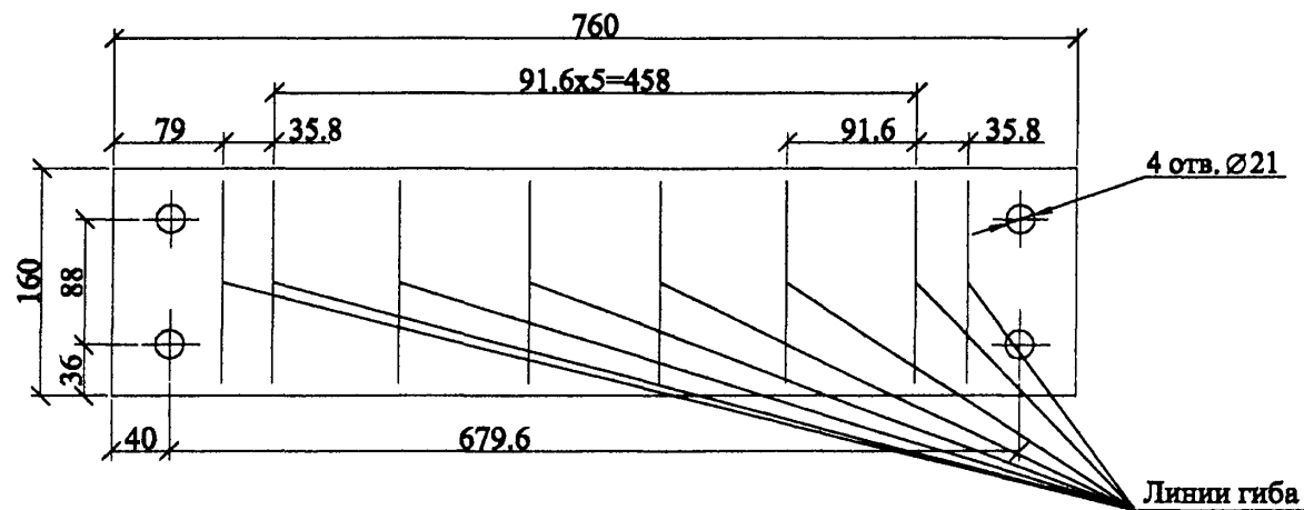
Развёртка поз. 4
