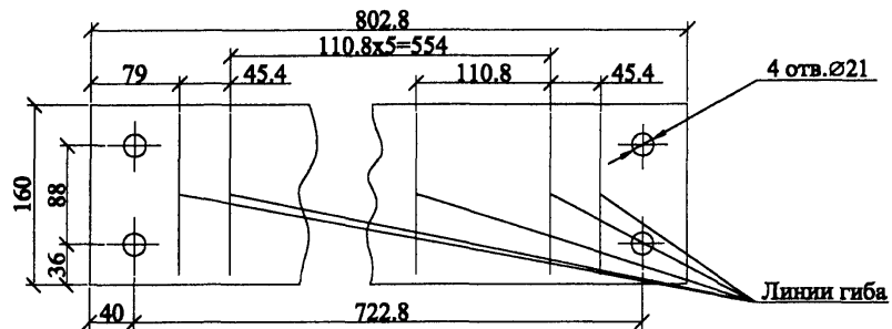
Развёртка поз.3
