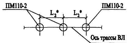
Схема установки стойки опоры
