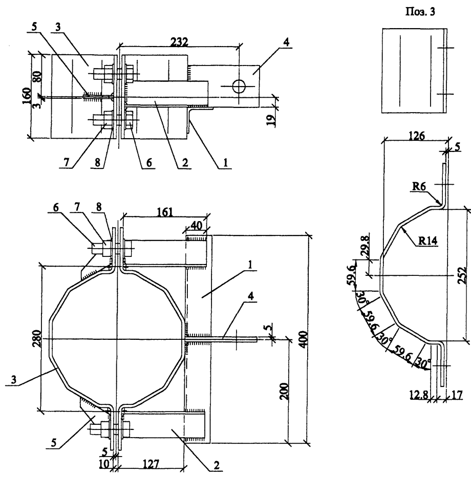
Развёртка поз. 3
