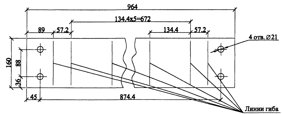
Развёртка поз. 1
