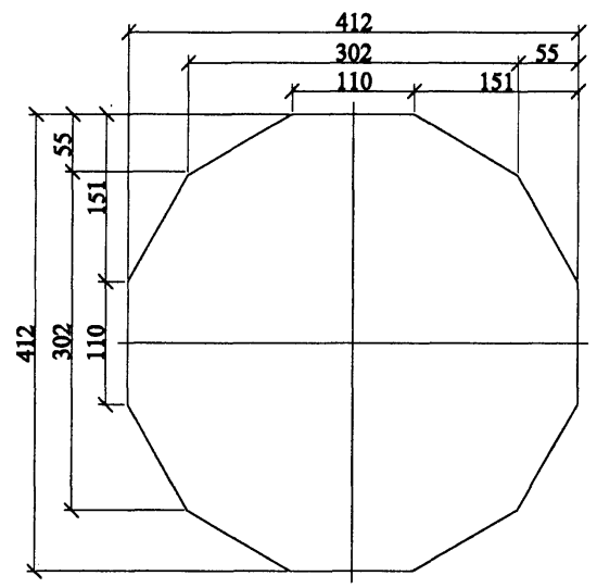
Поз. 1
