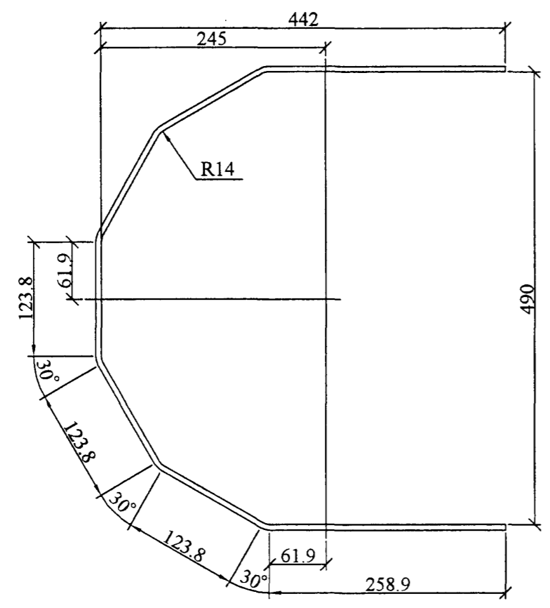
Поз. 1
