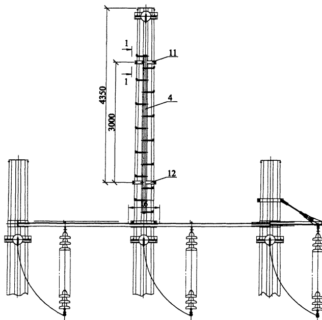
Схема 3 Опора АМ110-1 и УАМ110-1
