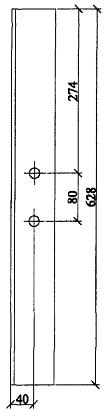
Поз. 2
