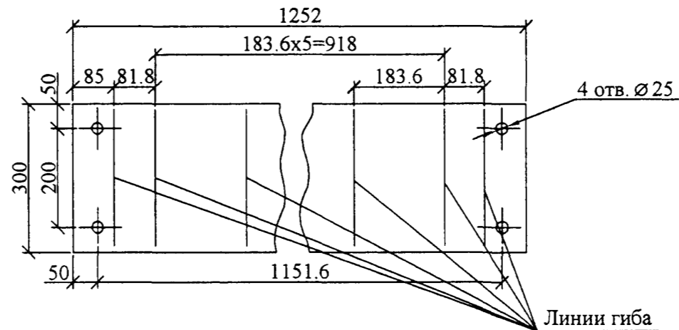
Развёртка поз. 1
