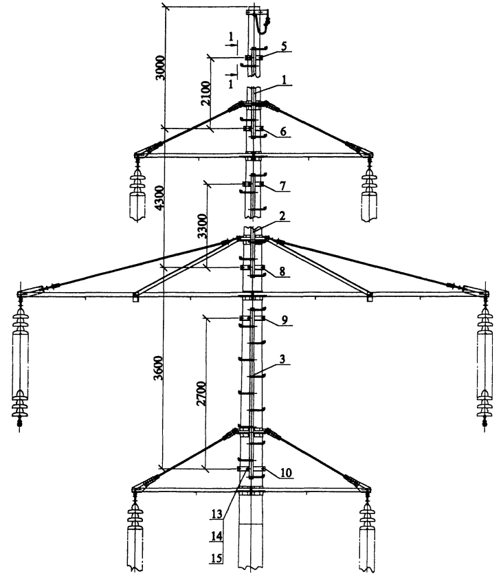
Схема 2 Опора ПМ110-2
