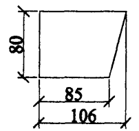
Поз. 7
