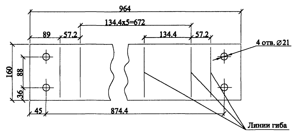
Развёртка поз. 6
