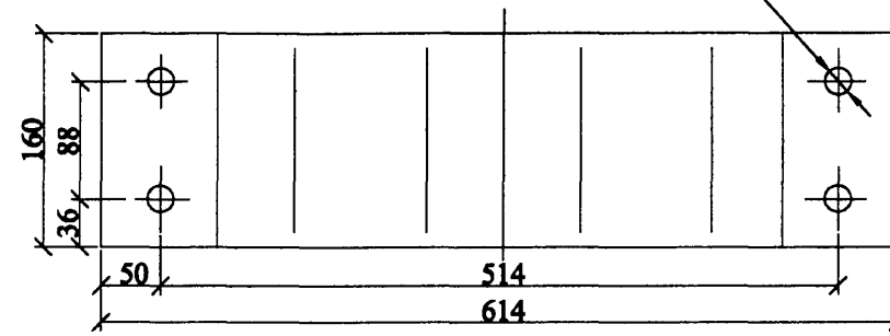
4 отв. Ø21
