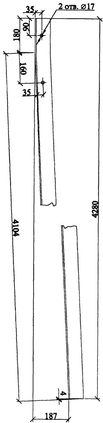
Поз. 1
