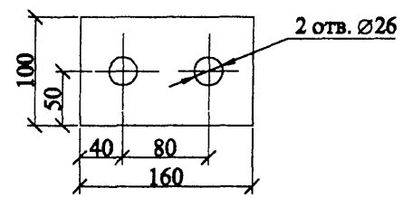
Поз. 8
